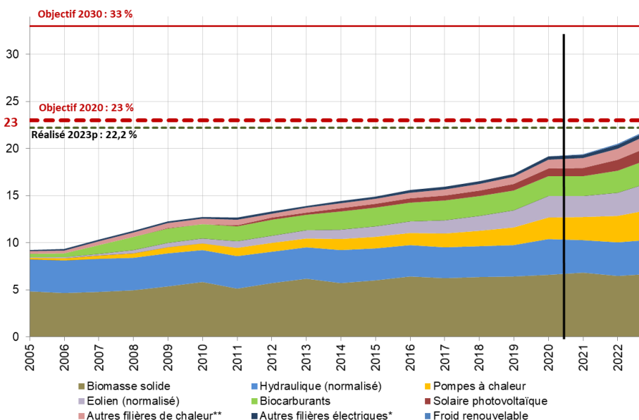
GRAPHIQUE 3 : PART DES ENR DANS LA CONSOMMATION FINALE BRUTE D'ÉNERGIE PAR FILIÈRE ET OBJECTIFS 2020 ET 2030
