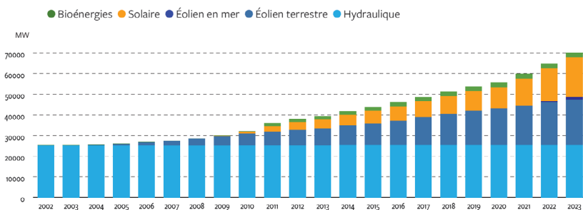
GRAPHIQUE 5 : EVOLUTION DE LA PUISSANCE INSTALLÉE 356
